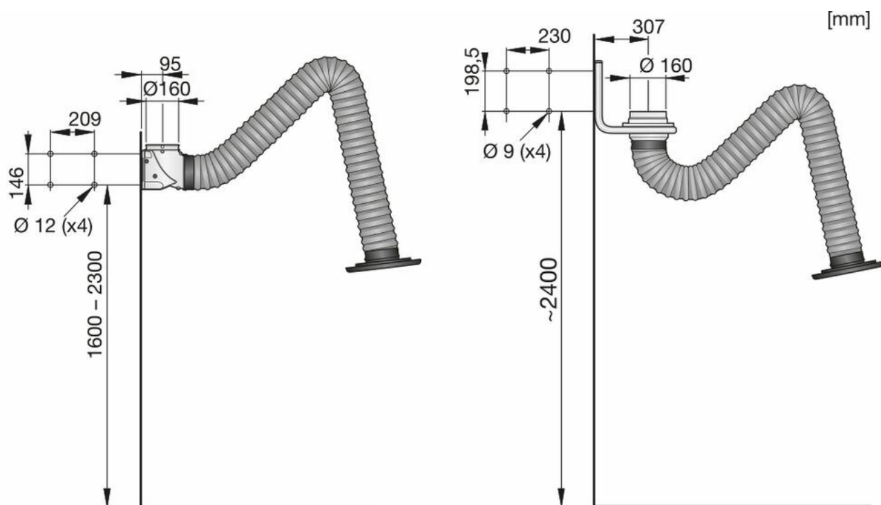
Vänster: Standardarm 2 & 3m. Höger: Standardarm 4 m.
